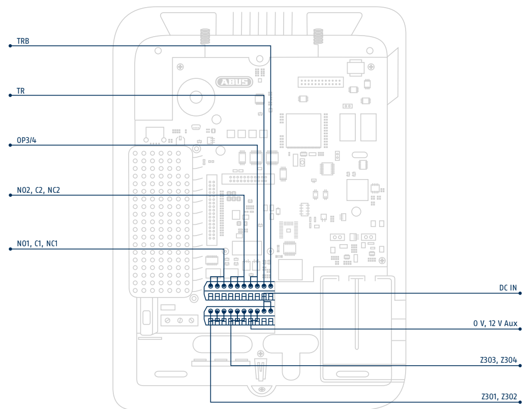
N01, C1, NC1 – relaisuitgang 1: potentiaalvrij relaiscontact, 24 VAC / 500 mA · N02, C2, NC2 – relaisuitgang 2: potentiaalvrij relaiscontact, 24 VAC / 500 mA · OP3/4 – transistoruitgangen: voor een bekabelde sirene, flitslicht en akoestisch alarm TR – Tamper Return: sabotage-ingang van een bekabelde sirene · TRB – Trouble: storingsmeldingsingang van een bekabelde sirene · Z301, Z302: bekabelde zones 301 en 302 · Z303, Z304: bekabelde zones 303 en 304 · 0 V, 12 V Aux: spanningsuitgang 13,8 V · DC IN 13,8 V +: aansluiting voedingsspanning 13,8 V
