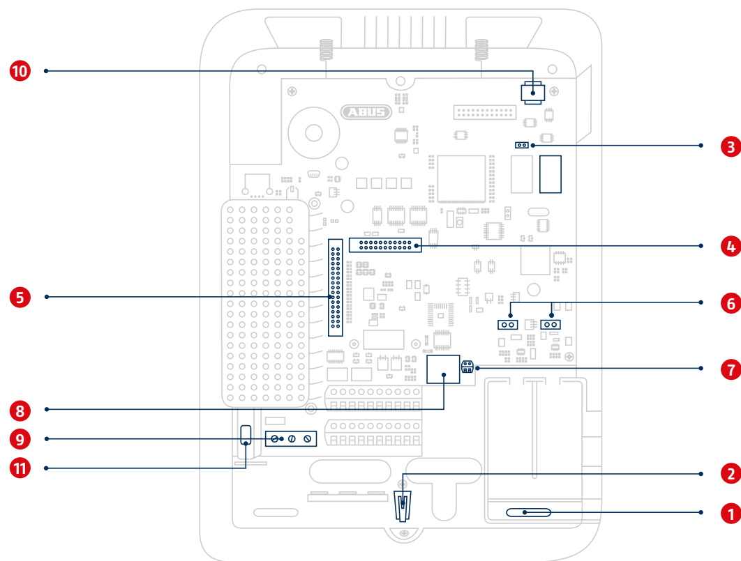
1. Bevestigingsopening voor schroeven · 2. Behuizing-sabotageschakelaar · 3. Code Reset Pins · 4. Aansluiting voor optionele gsm-module · 5. Aansluiting van flatcable · 6. Aansluitingen voor accupack · 7. Analoge telefoonaansluiting · 8. Aansluiting voor LAN-kabel · 9. Aansluiting netspanning 110 V/230 V AC 50/60 Hz · 10. SD-kaarthouder · 11. Zekeringhouder netzekering
